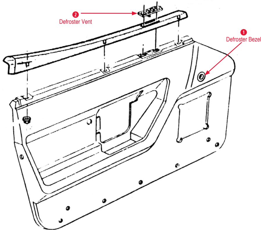
1 Defroster Bezel
